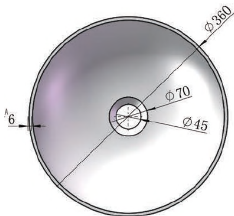
Grundriss
