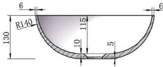
Längsschnitt
